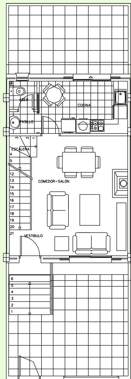
PLANTA BAJA
